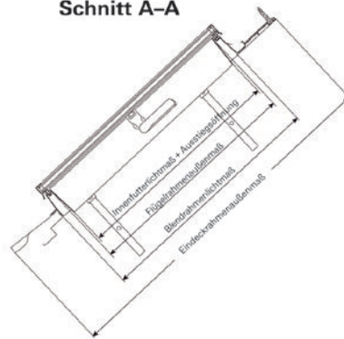
Schnitt A-A
