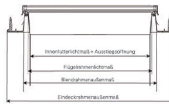
Schnitt B-B
