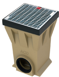
Hofablauf aus Polymerbeton mit Maschenrost (Stahl verzinkt, MW 31x17 mm) und Gusszarge
