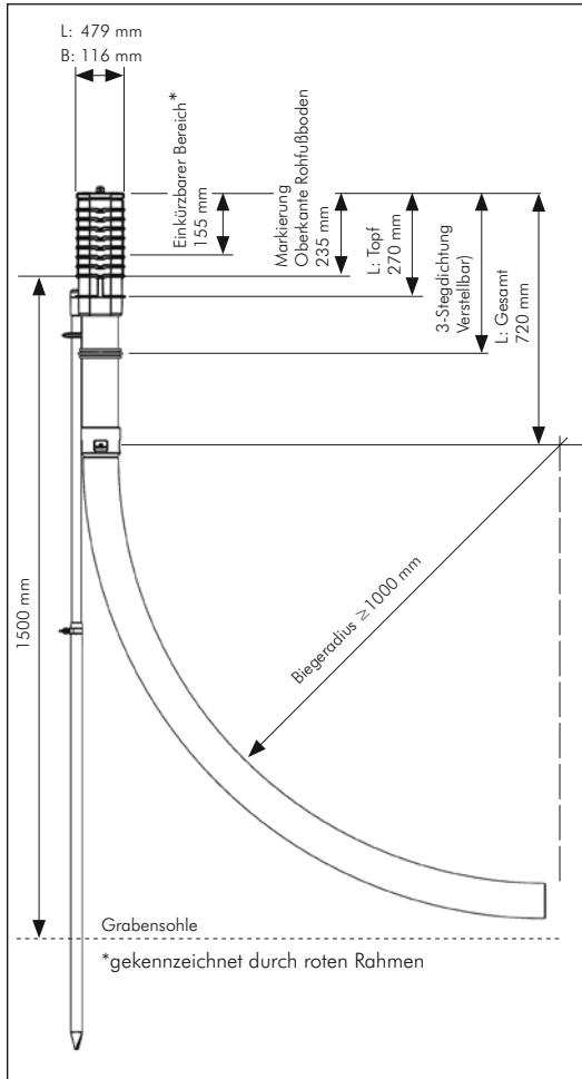
Vermassung des Rohbauteils
