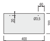
Format 40 x 20 cm, vollkantig, gelocht
