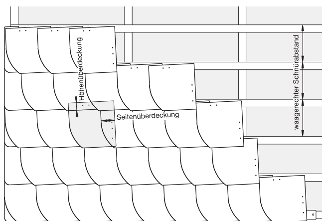
Beispiel: Format 30 x 30 cm, Bogenschnitt links, mit eingebundenem Anfangort
