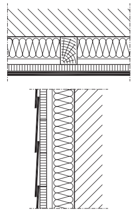
Schalung auf senkrechter Grundlattung
