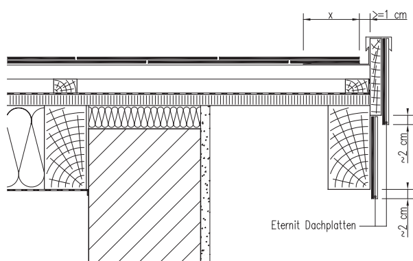
Ortgangausbildung mit hochstehender Ortblende
