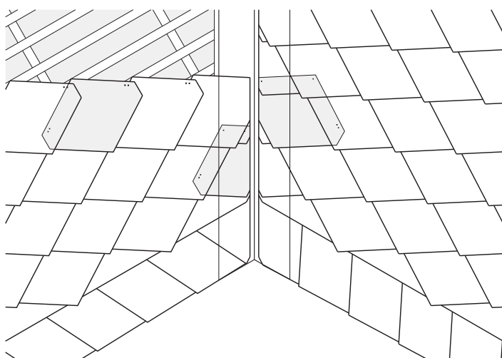
Blechkehle bei Rhombusdeckung Format 40 x 44 cm
