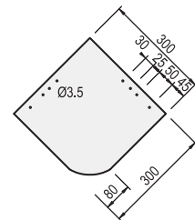
30 x 30 cm, gerundet
