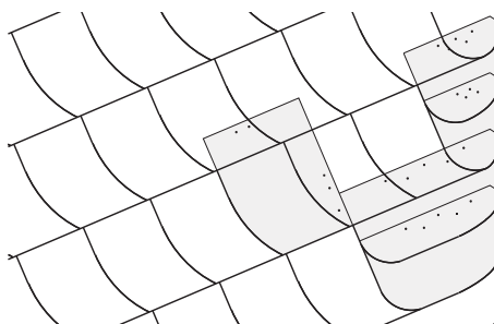
Ortgangausbildung als Doppelendort
