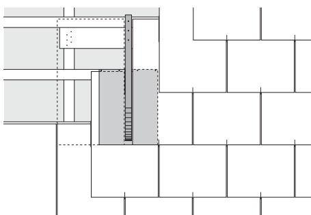
Dachhaken bei Doppeldeckung 32 x 60 cm
