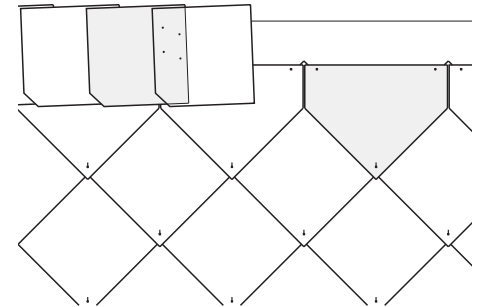
Firstausbildung mit Ausspitzerplatten und Firstgebinde, Format 30 x 30 cm
