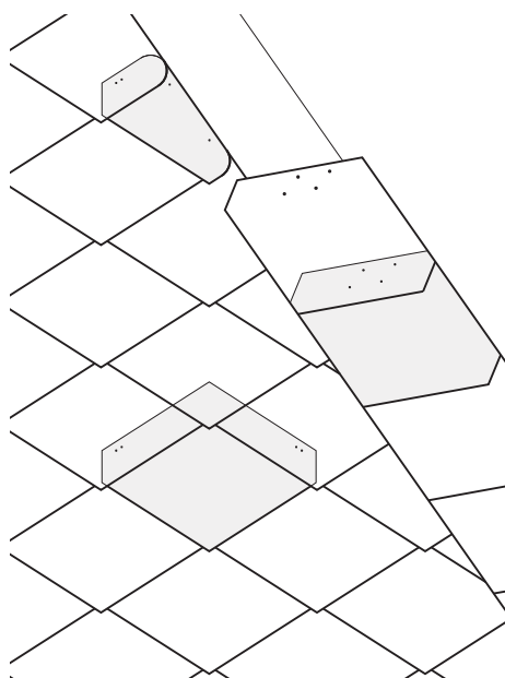
Rhombusdeckung mit aufgelegtem Gebinde
