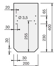
20 x 40 cm, gestutzt
