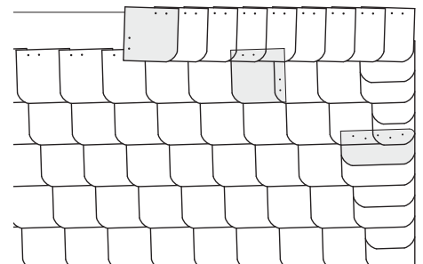
Oberer Abschluss mit aufgelegtem Abschlussgebände und Doppelort
