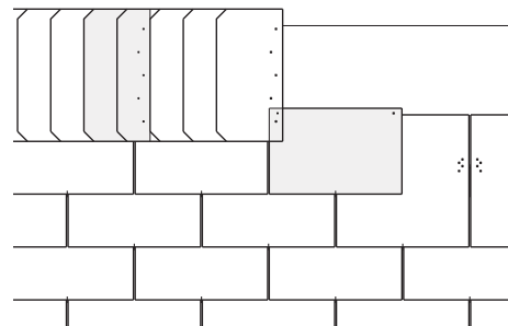
Firstausbildung mit Firstgebinde, Format 40 x 20
