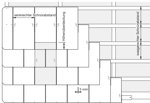
Beispiel: Format 30 x 60 cm, vollkantig
