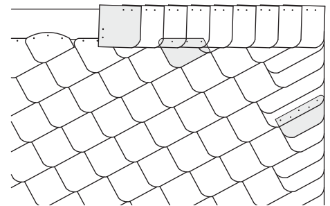
Oberer Abschluss mit aufgelegtem Abschlussgebinde und Doppelendort
