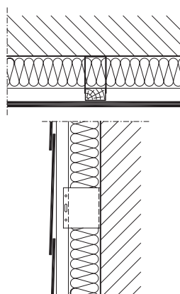
Aluminium-U-Halter mit senkrechter Traglattung
