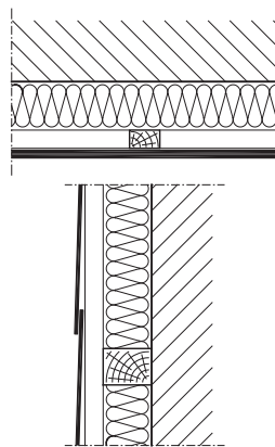
Senkrechte Traglattung auf waagerechter Grundlattung
