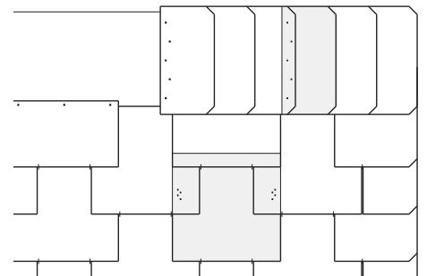
Oberer Abschluss mit aufgelegtem Abschlussgebinde, Format 40 x 20 cm
