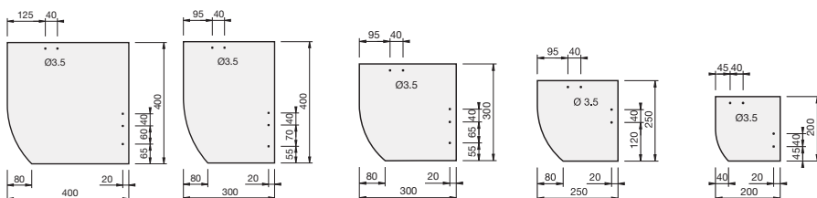
40 x 40 cm, Bogenschnitt 30 x 40 cm, Bogenschnitt 30 x 30 cm, Bogenschnitt 25 x 25 cm, Bogenschnitt 20 x 20 cm, Bogenschnitt
