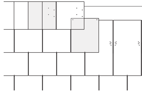
Firstausbildung mit Firstgebinde, Format 30 x 30
